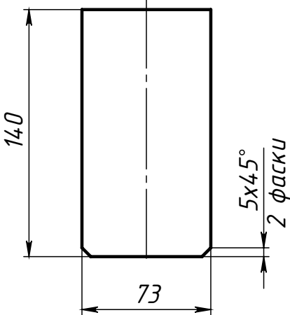
Поз.3 (Ребро среднее)
