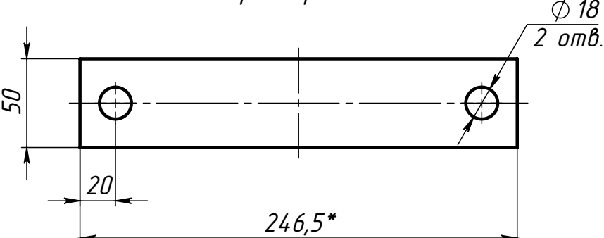
Поз.4 (Полухомут) развертка
